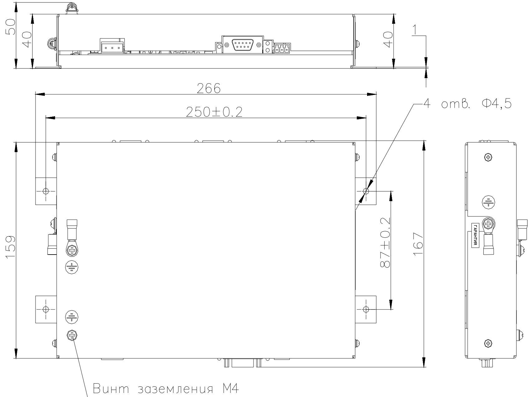
1. Размеры для справок
