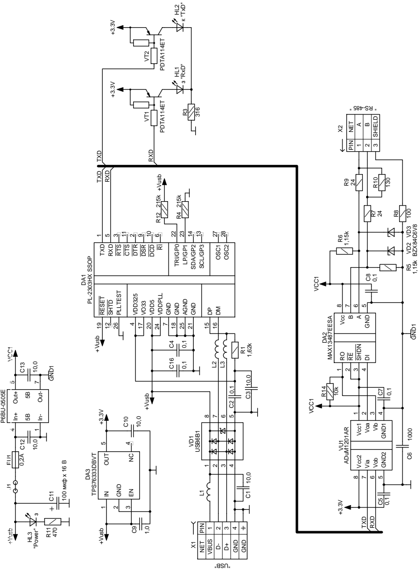
Приложение А Схема электрическая принципиальная блока сопряжения "Топаз-119-26М" ДСМК.687242.143 [5]
