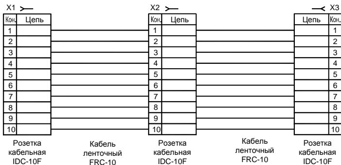
Кабель K2
