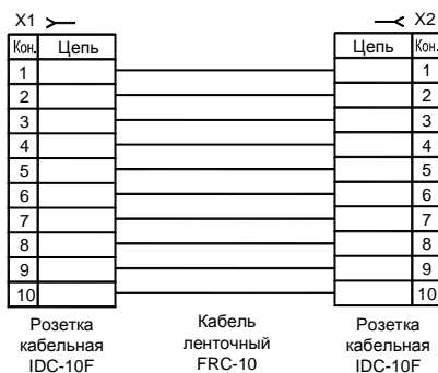
Кабель K1
